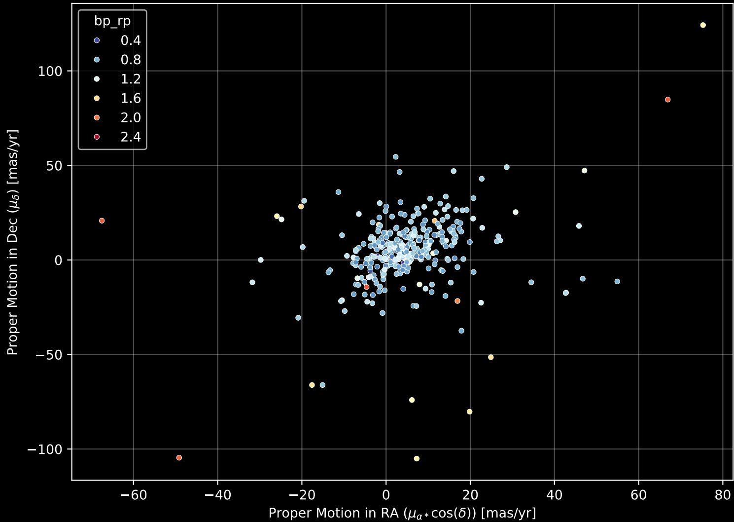
GALAH DR4 Field: [217] Proper Motion Diagram (n= 331)
