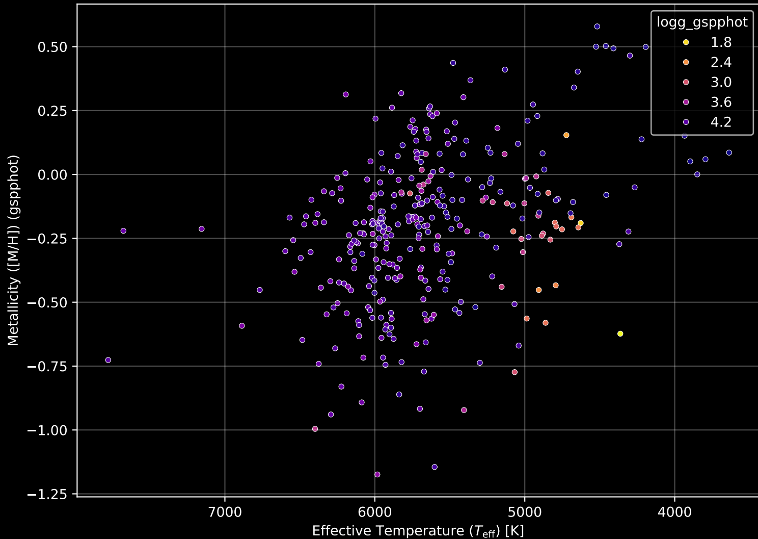
GALAH DR4 Field: [217] Stellar Population Parameters (n= 331)
