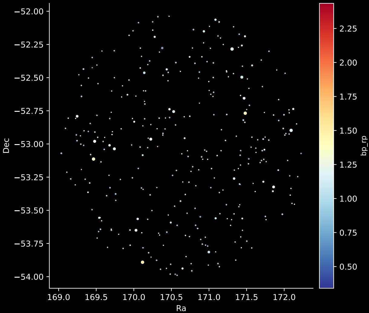
GALAH DR4 Field: [217] Stars: 331
