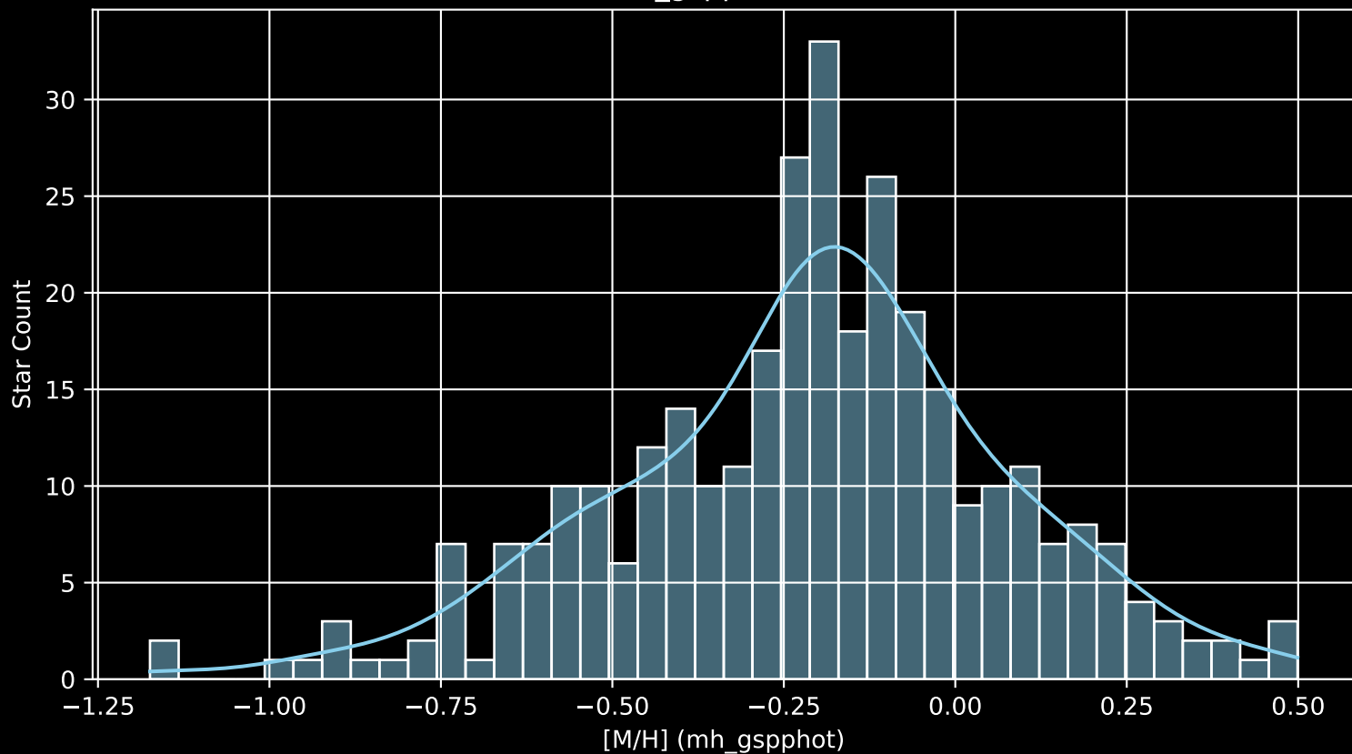
GALAH DR4 Field: [217] [M/H] (mh_gspphot) (n= 328)
