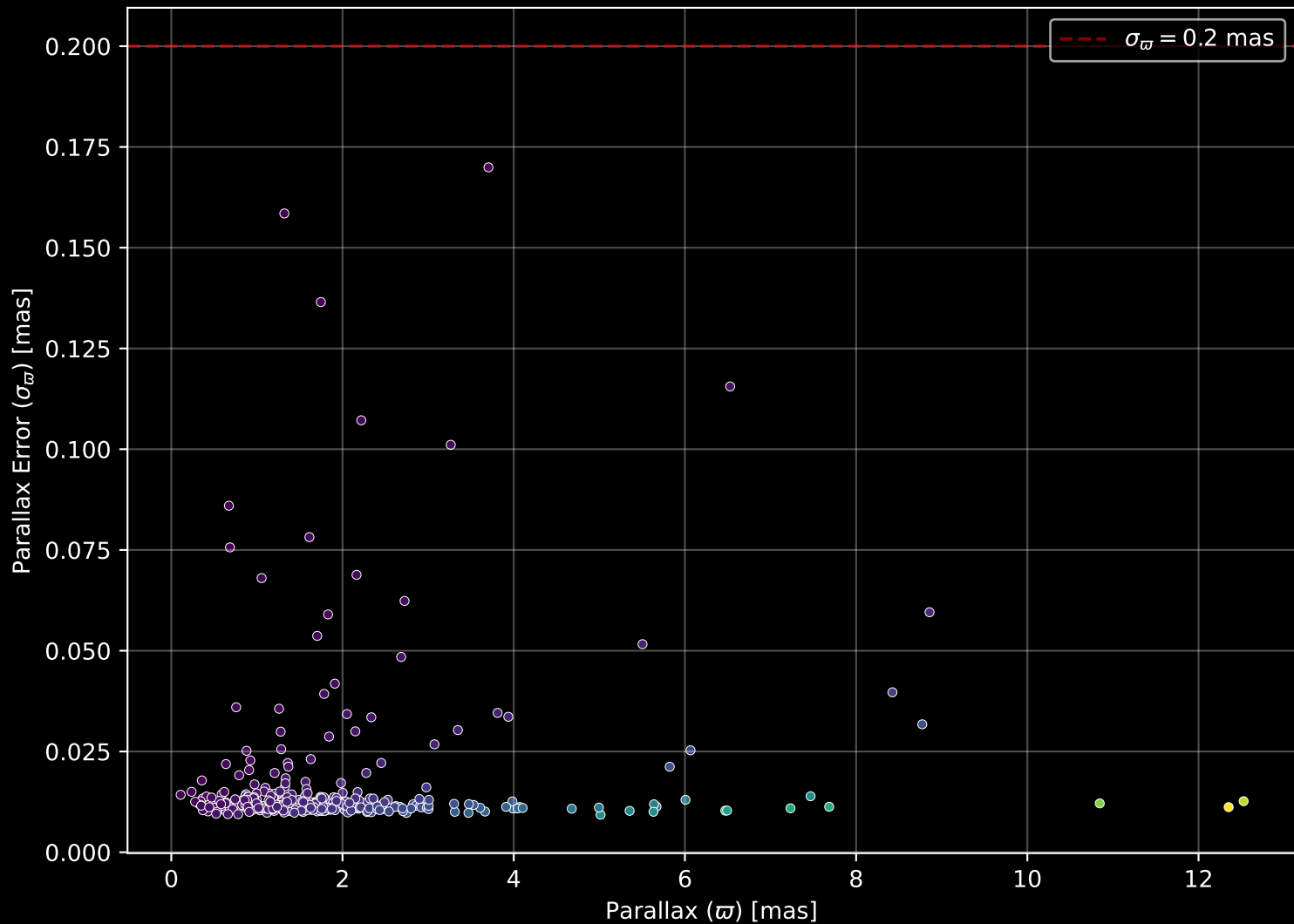
GALAH DR4 Field: [217] Parallax Quality (n= 331)
